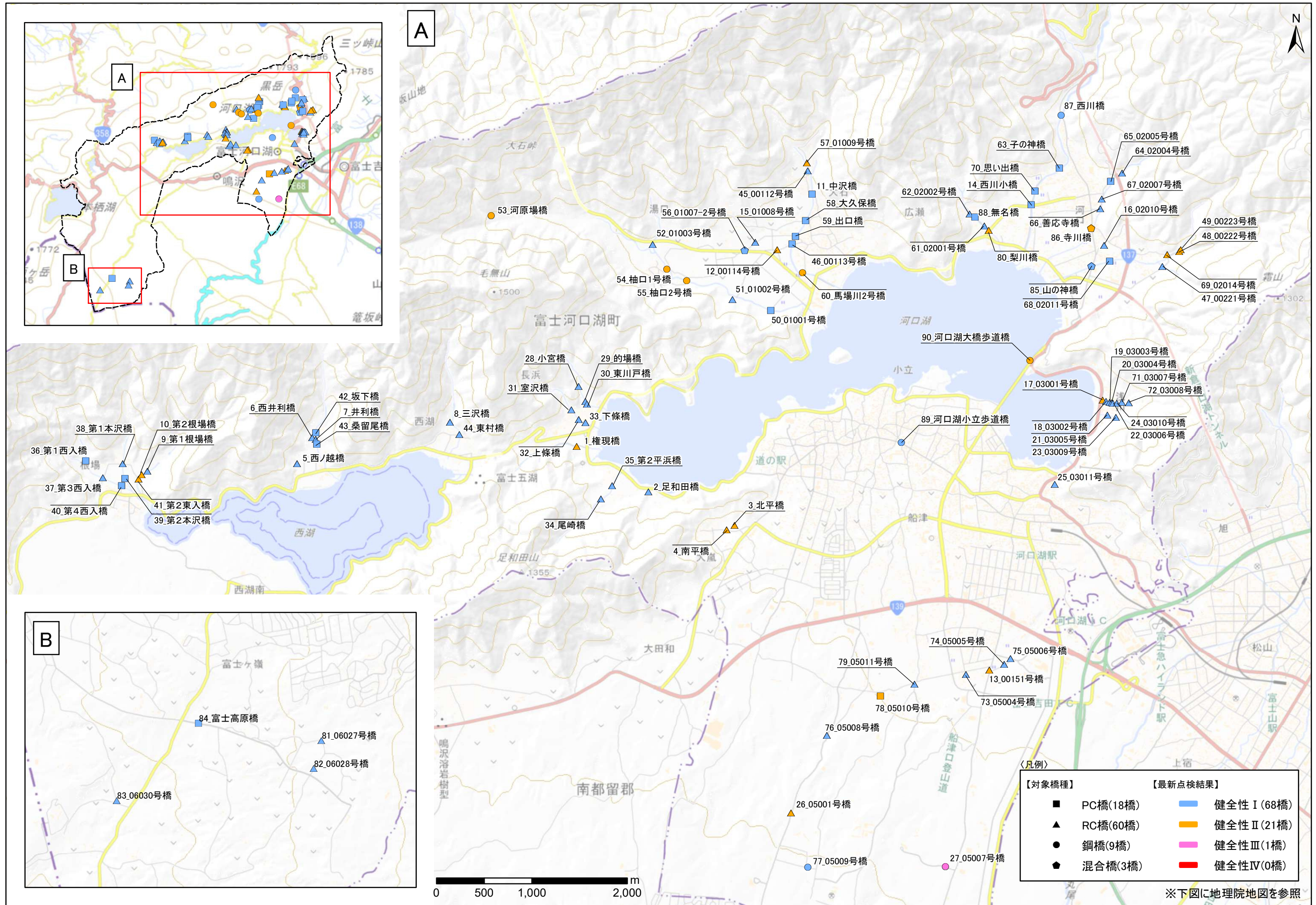
図2.2 橋梁位置図
